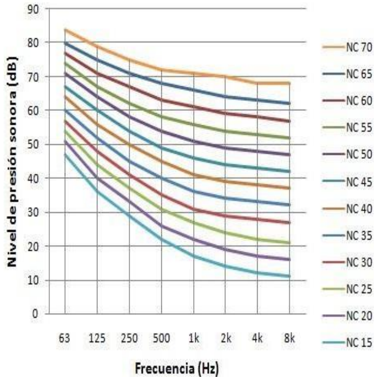
GRÁFICA X.2.- CURVAS NC
